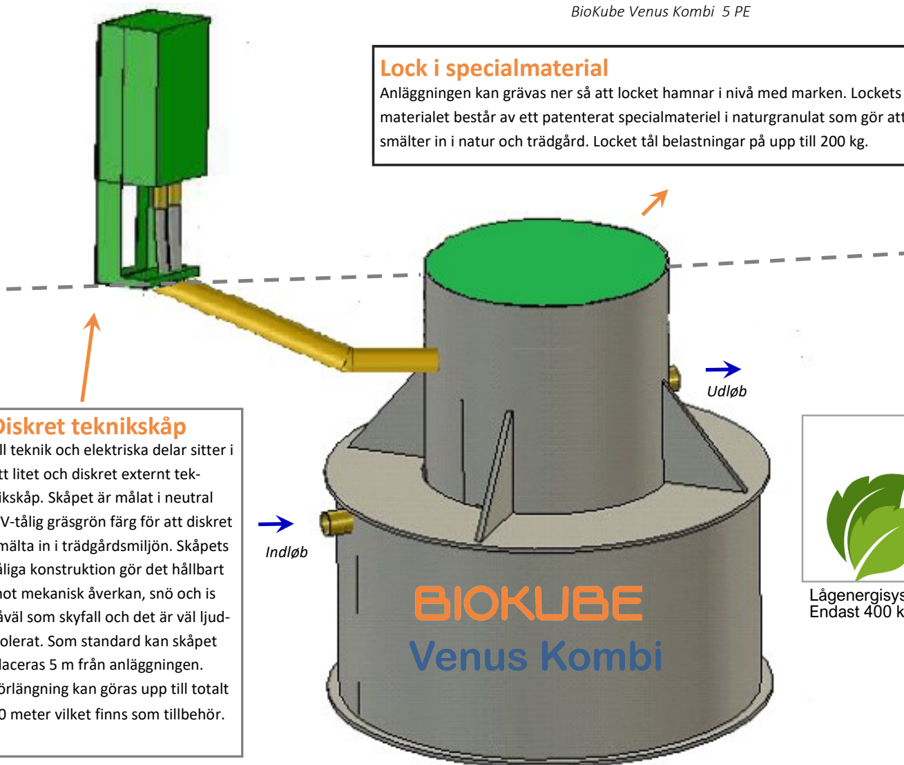
BioKube Venus Kombi 5 PE
